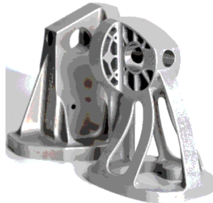
Şekil 4: Toz Yataklı Metal Katmanlı İmalat Örnekleri
