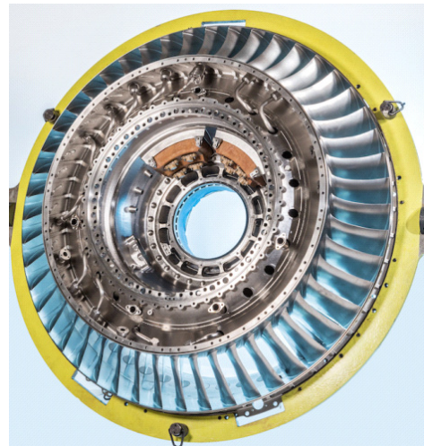
Şekil 19: Rolls Royce Trent XWB motoru “Front Bearing Housing” parçası
