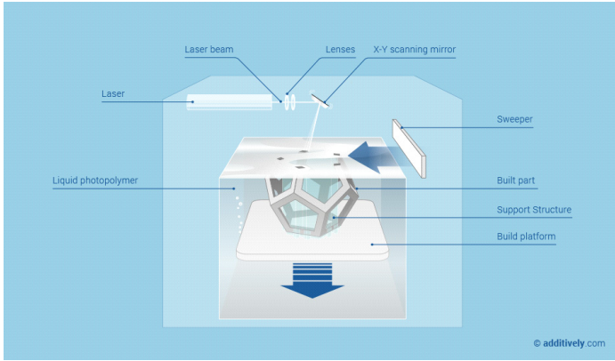
Şekil 10: Stereolithografi uygulaması
