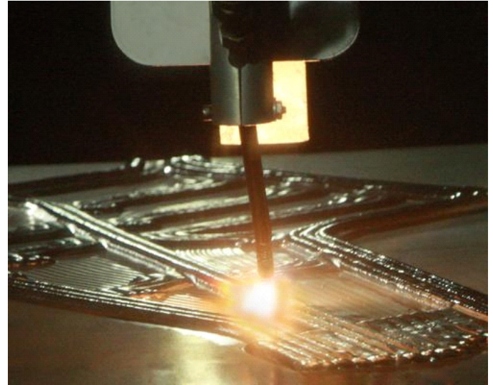
Şekil 7: Elektron kaynağı
