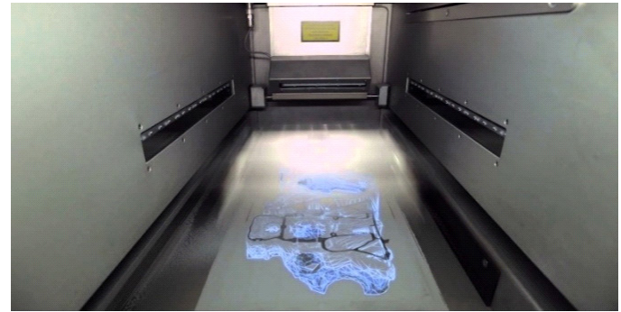
Şekil 3: Toz yataklı lazer eritme sistemleri
