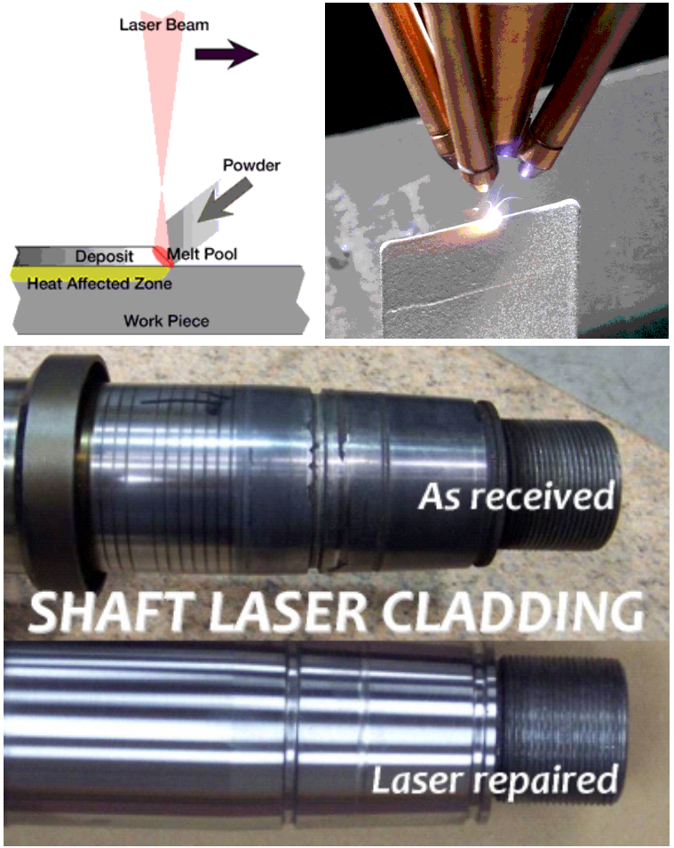
Şekil 3: Toz yataklı lazer eritme sistemleri
